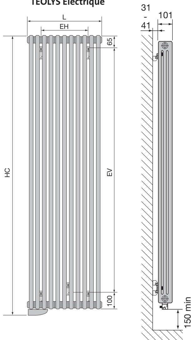
Electric COLUMN TÉOLYS Électrique
