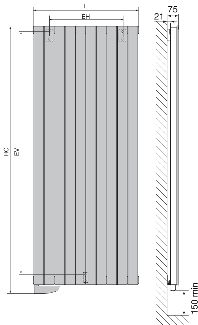
Electric DÉCOR CHORUS Électrique
