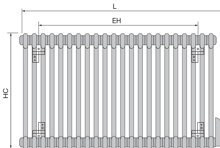
Electric COLUMN TÉOLYS Électrique
